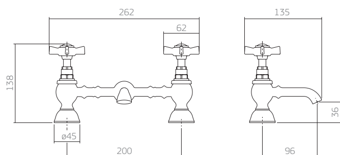
1875.C67.EXT misturador lavatório mesa
