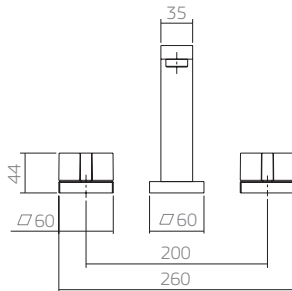
1877.C88 misturador lavatório mesa
