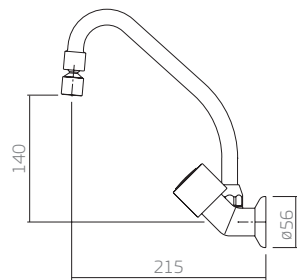
1168.C40.CR torneira cozinha parede bica móvel
