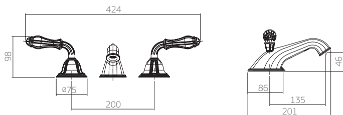
1875.C81.P misturador lavatório mesa com pop-up
