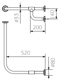
2380.E.BR barra de canto para lavatório
