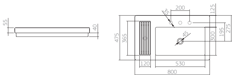
L.1044C cuba com saboneteira grelha
