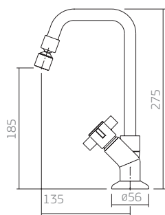
1167.C46 torneira cozinha mesa bica móvel
