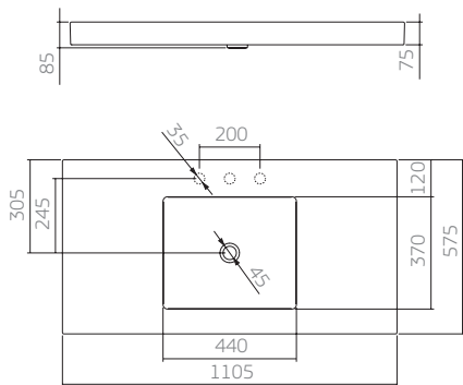
L.117 cuba retangular de apoio
