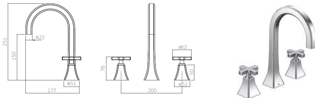
1877.C.WSH misturador lavatório mesa
