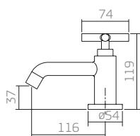
1197.C64 torneira lavatório mesa
