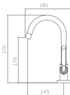
1198.C61 torneira lavatório mesa
