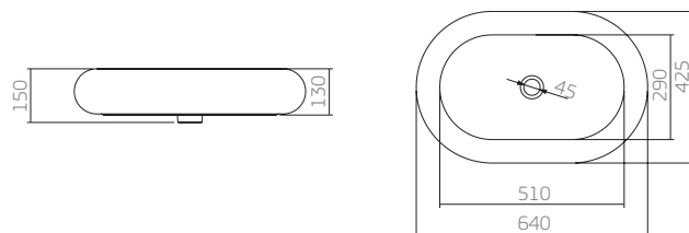
L.1035 cuba de apoio oblonga
