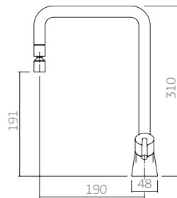
1167.C73 torneira cozinha mesa bica móvel
