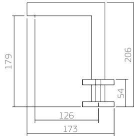
1877.C85 misturador lavatório mesa
