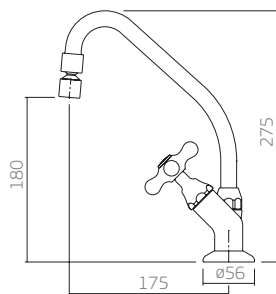
1167.C52 torneira cozinha mesa bica móvel
