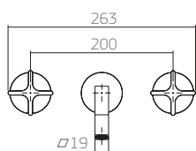
1878.C.STR misturador lavatório parede
