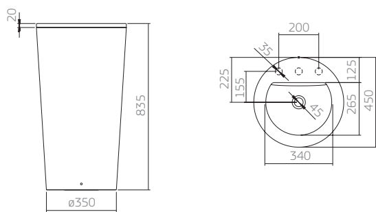
LC.1272* cuba de piso cilíndrica com mesa
