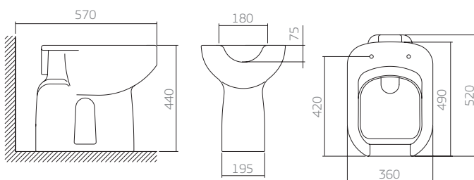
AP.52 assento com abertura frontal
