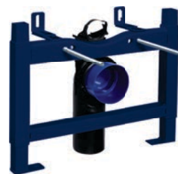
1100.SP.133 suporte para instalação para bacia em drywall
