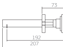
1878.C85 misturador lavatório parede
