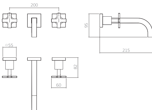
1878.C.CLN misturador lavatório parede
