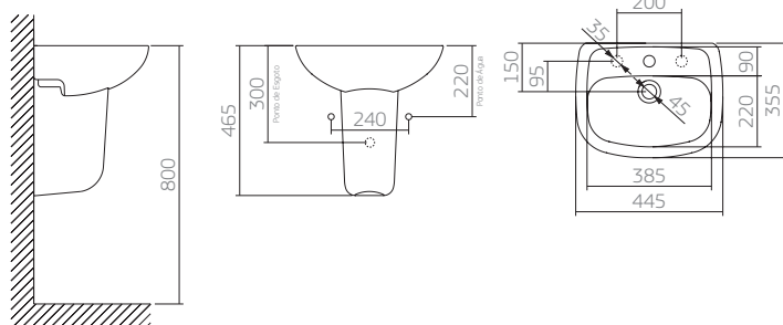
C.510 (coluna suspensa) lavatório pequeno com coluna suspensa
