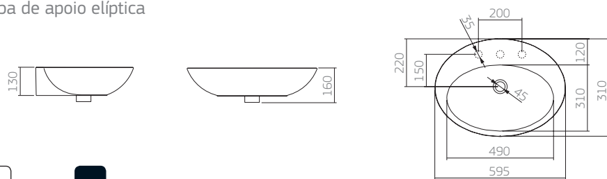
L.1038 cuba de apoio elíptica
