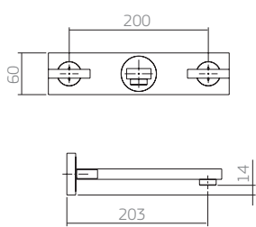
1878.C87 misturador lavatório parede
