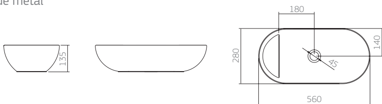
L.1060C cuba de apoio com saboneteira de metal
