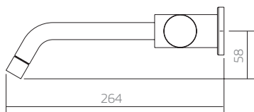
1178.C35 torneira lavatório parede
