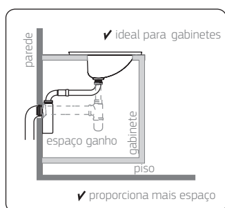
1682.C.112 sifão articulado para cozinha
