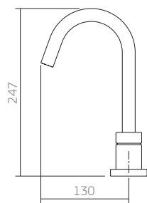
1191.C86 torneira lavatório mesa
