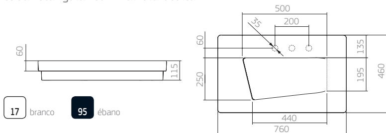
L.89 cuba retangular com válvula oculta
