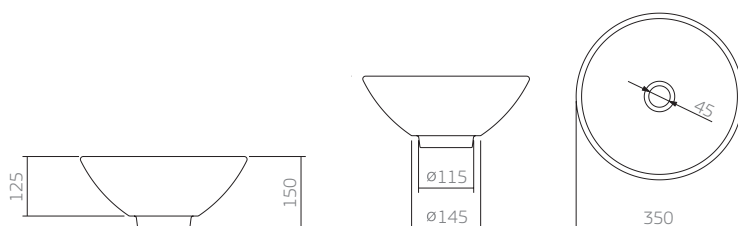
L.155 cuba de apoio redonda
