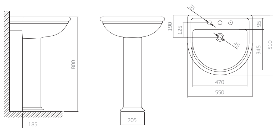
L.2 (lavatório) C.2 (coluna) lavatório com coluna
