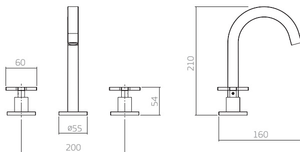
1877.C.CLN misturador lavatório mesa
