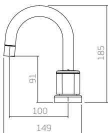
1877.C43 misturador lavatório mesa
