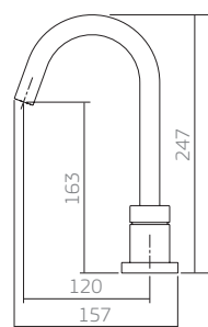
1877.C86 misturador lavatório mesa
