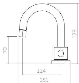
1877.C35 misturador lavatório mesa
