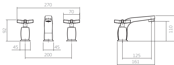
1875.C89 misturador lavatório mesa
