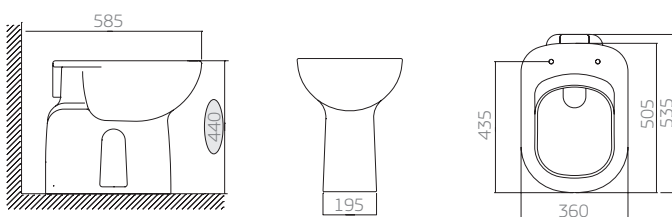
P.510 bacia vogue plus conforto sem abertura frontal
