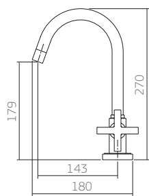
1198.C64 torneira lavatório mesa
