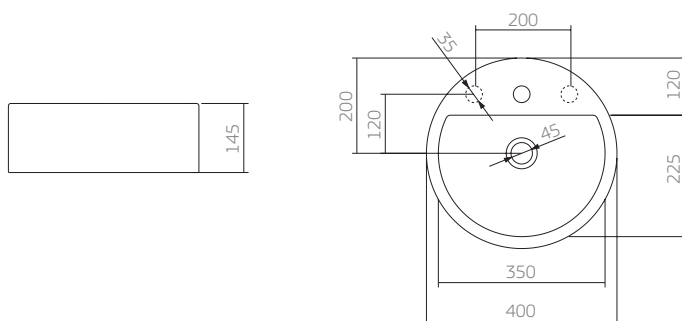
L.71C** cuba cilíndrica suspensa com porta- toalha cromado
