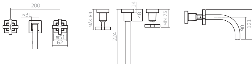
1878.C94 misturador lavatório parede
