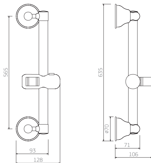
1980.C barra deslizante Belle Époque
