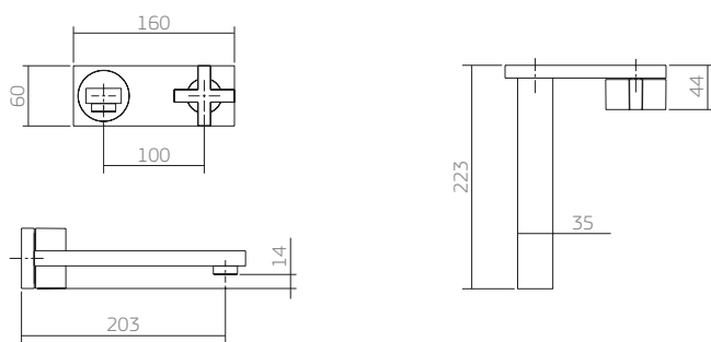
1179.C88 torneira lavatório embutida parede
