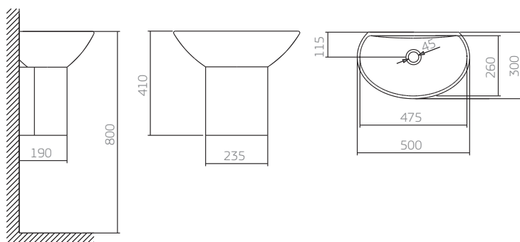
L.69 cuba de apoio parede oval + C.69 coluna suspensa para L.69
