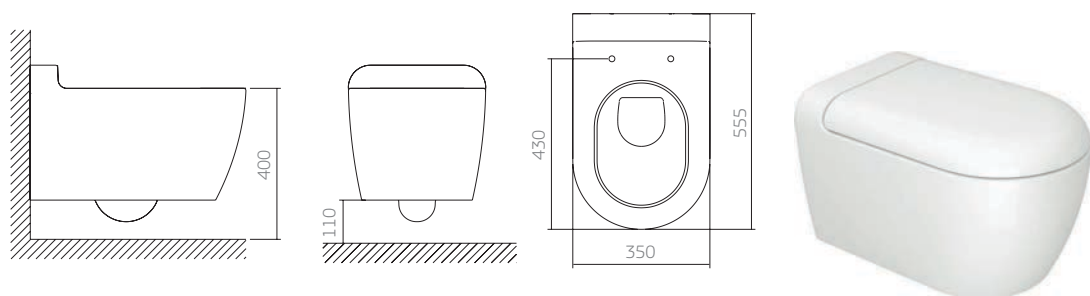
P.192 bacia convencional suspensa
