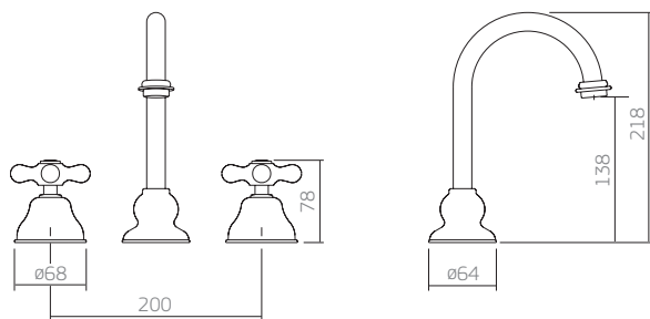
1877.C52 misturador lavatório mesa
