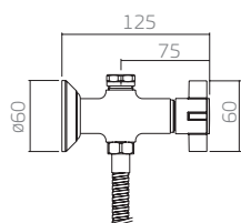
1984.C46.ACT.BR ducha higiênica com registro, derivação e gatilho branco
