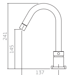
1877.C72 misturador lavatório mesa
