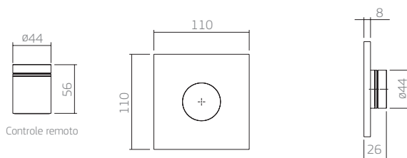
2993.C.TCH.CON monocomando para chuveiro, com controle remoto alta pressão
