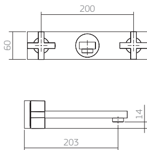
1878.C88 misturador lavatório parede
