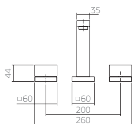
1877.C87 misturador lavatório mesa
