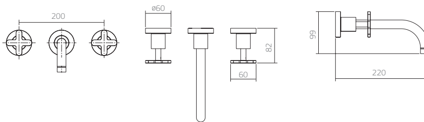
1878.C.DSC misturador lavatório parede
