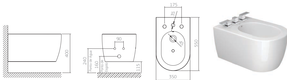
B.192 bidê suspenso (3 furos)
