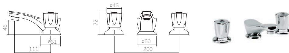
1875.C50 misturador lavatório mesa
