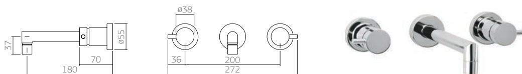
1878.C72 misturador lavatório parede
