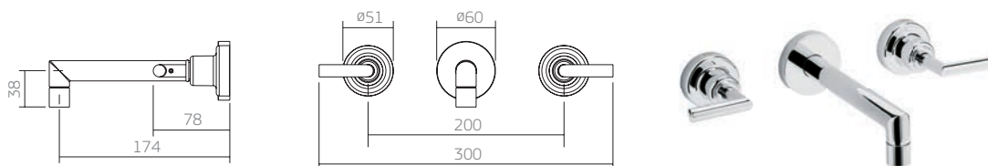
1878.C24 misturador lavatório parede
