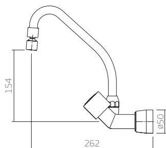
1258.C40.CR misturador cozinha parede bica móvel
