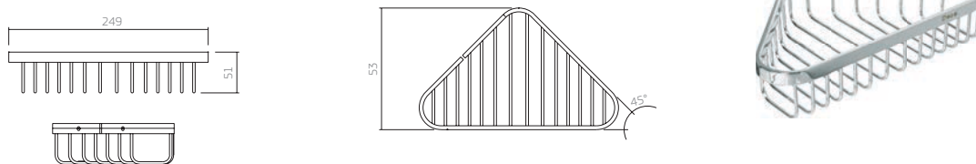
2072.C saboneteira triangular de canto
