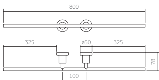
2042.C.SLM porta-toalha barra dupla
