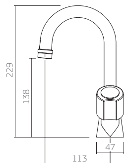
1195.C40.CR torneira lavatório mesa
