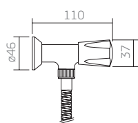
1984.C.ACT ducha higiênica com registro
