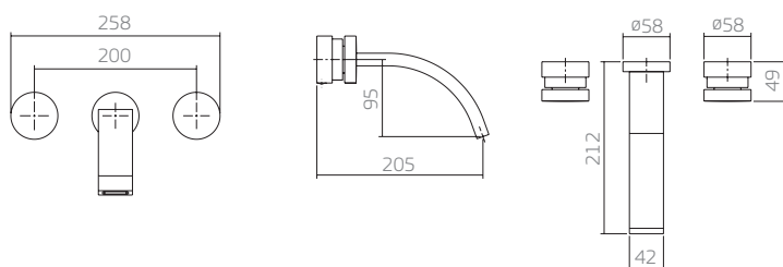
1878.C95 misturador lavatório parede
