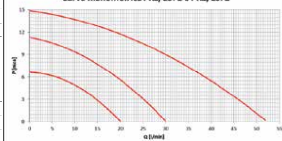
Curva manométrica PRZ/15F1 e PRZ/15F2
